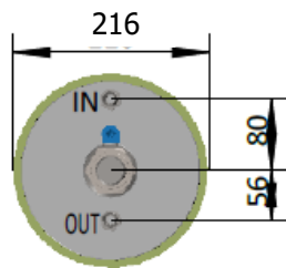
Bottom Flange
